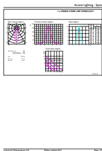
MASTER LEDspot PAR 60W E27 827 25D
